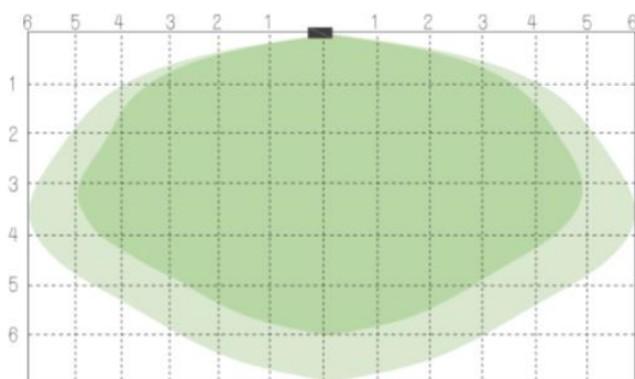
Montaggio a soffitto (m) Ceiling mounting (m)
